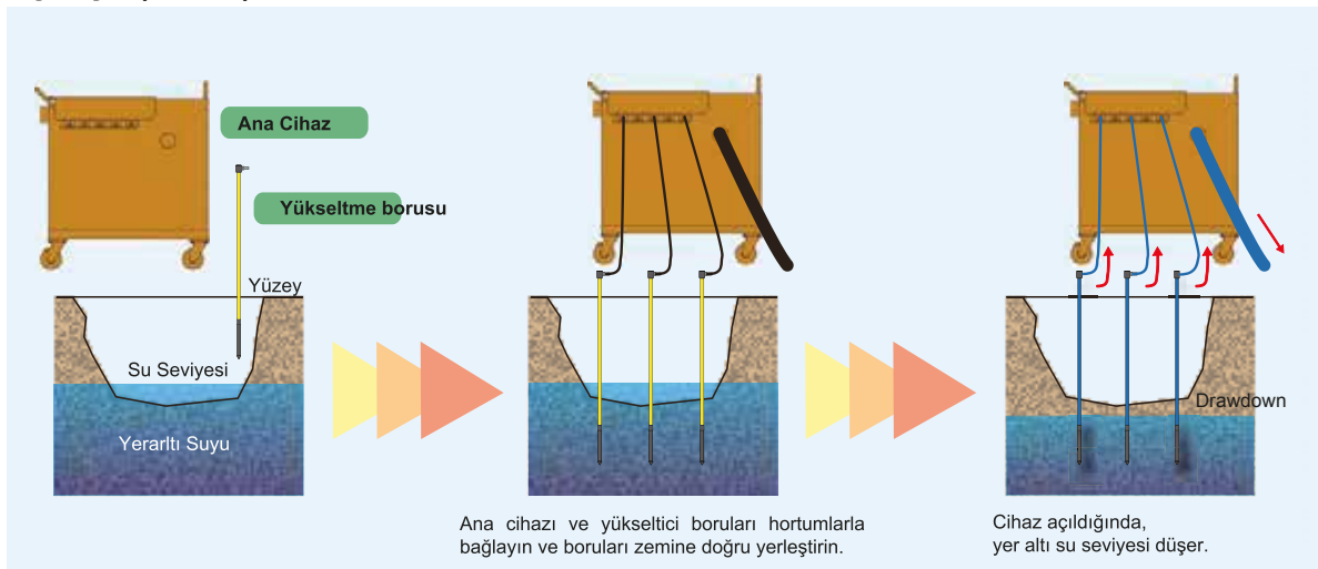
Yükseltme borusu
